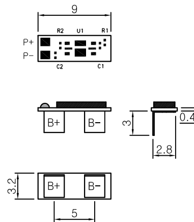
PCM(NOTE 4) SCALE:2/1
